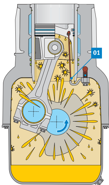
Fig. 2: Lubrifierea directă și indirectă a componentelor cu ulei injectat și centrifugat
